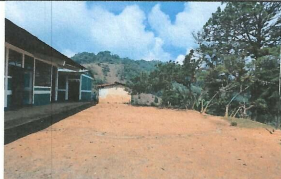
Foto 4: Se realizará el mejoramiento e instalación del techo con lámina troquelada para tener un mejor ambiente.
